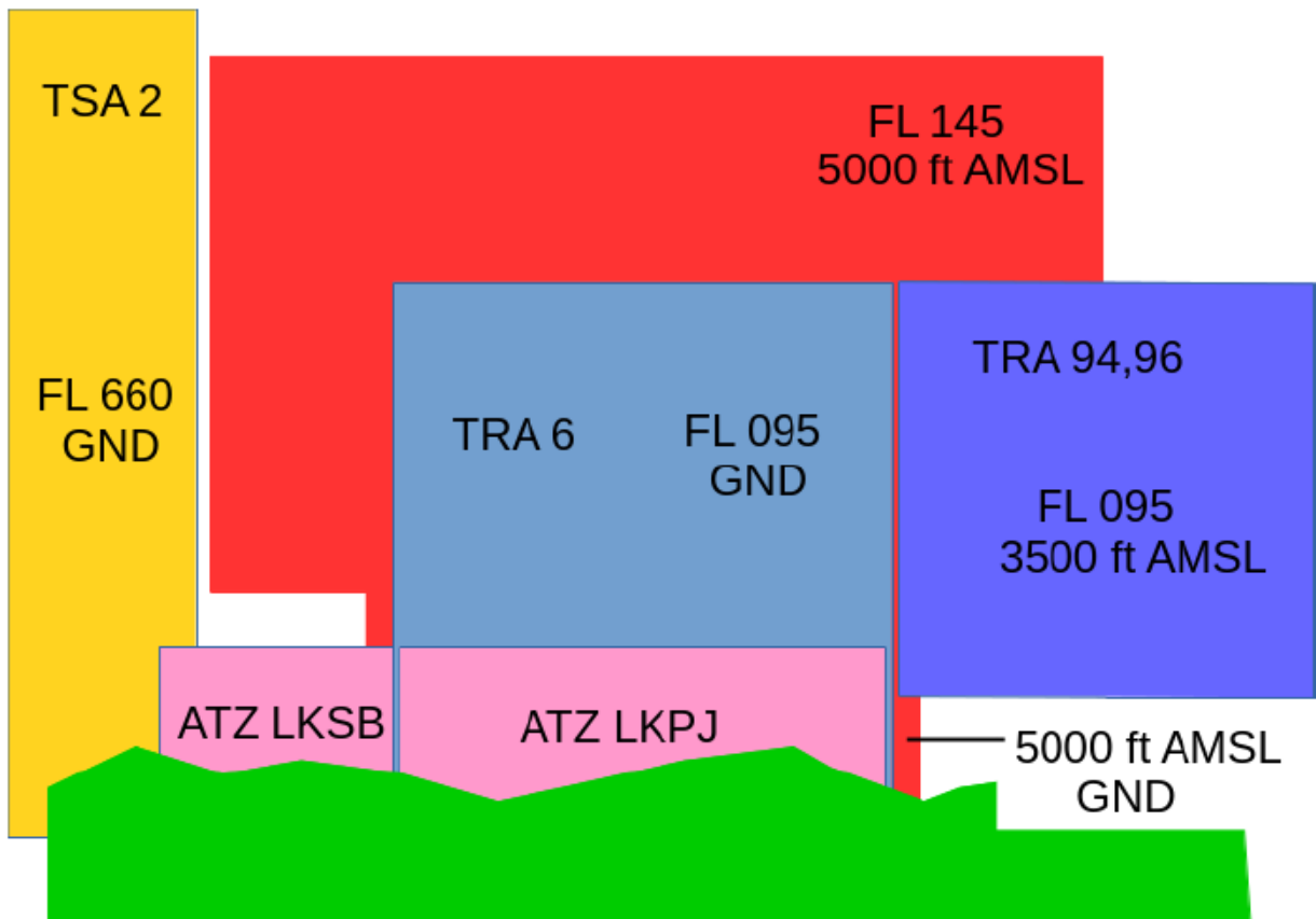
Obr. 2 – schéma vertikálního řezu, navrhovaný prostor zobrazen červeně.
