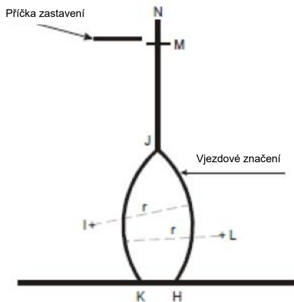
Obrázek 9 – Posunuté vjezdové značení příďového podvozku
