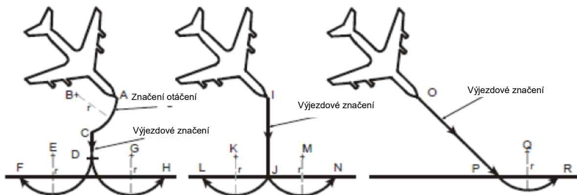
Obrázek 11 – Posunuté výjezdové značení předřadového podvozku
