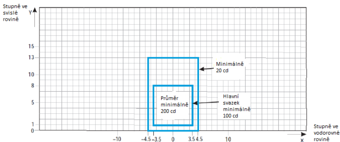
Obrázek U-17. Izokandelový diagram pro osová návěstidla pojezdové dráhy (rozstup 15 m), příček zákazu vstupu a stop příčky v přímých částech určený pro použití v podmínkách RVR nižší než o hodnotě 300 m
