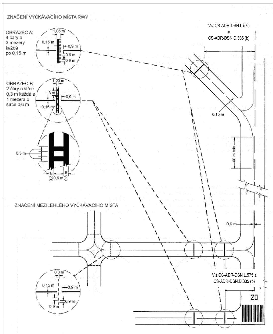
Obrázek L-5. Značení na jezdové dráze (spolu se základním značením RWY)
