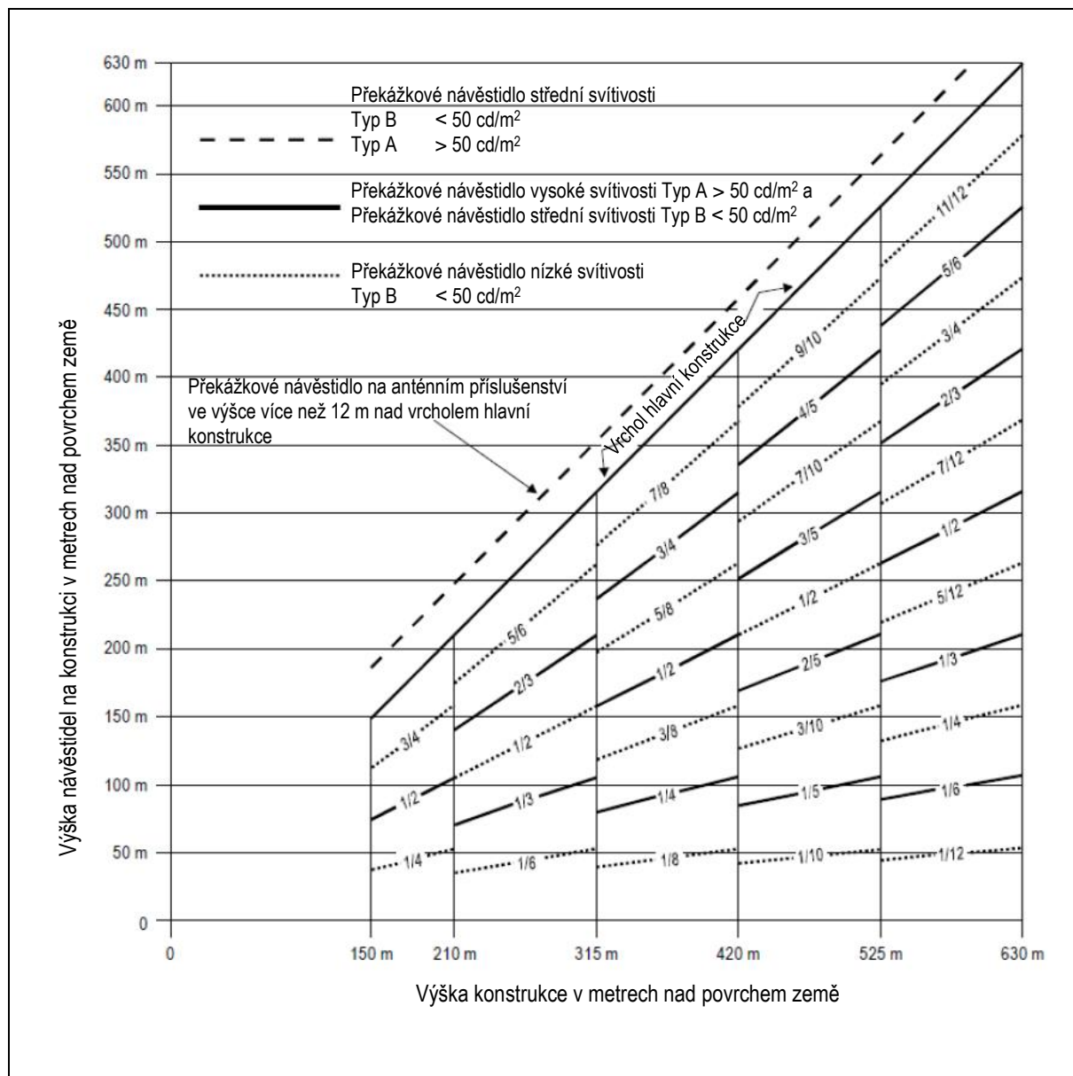
Obrázek GM-Q-7. Duální systém překážkových návěstídel vysoké/střední svítivosti typu A/typu B
