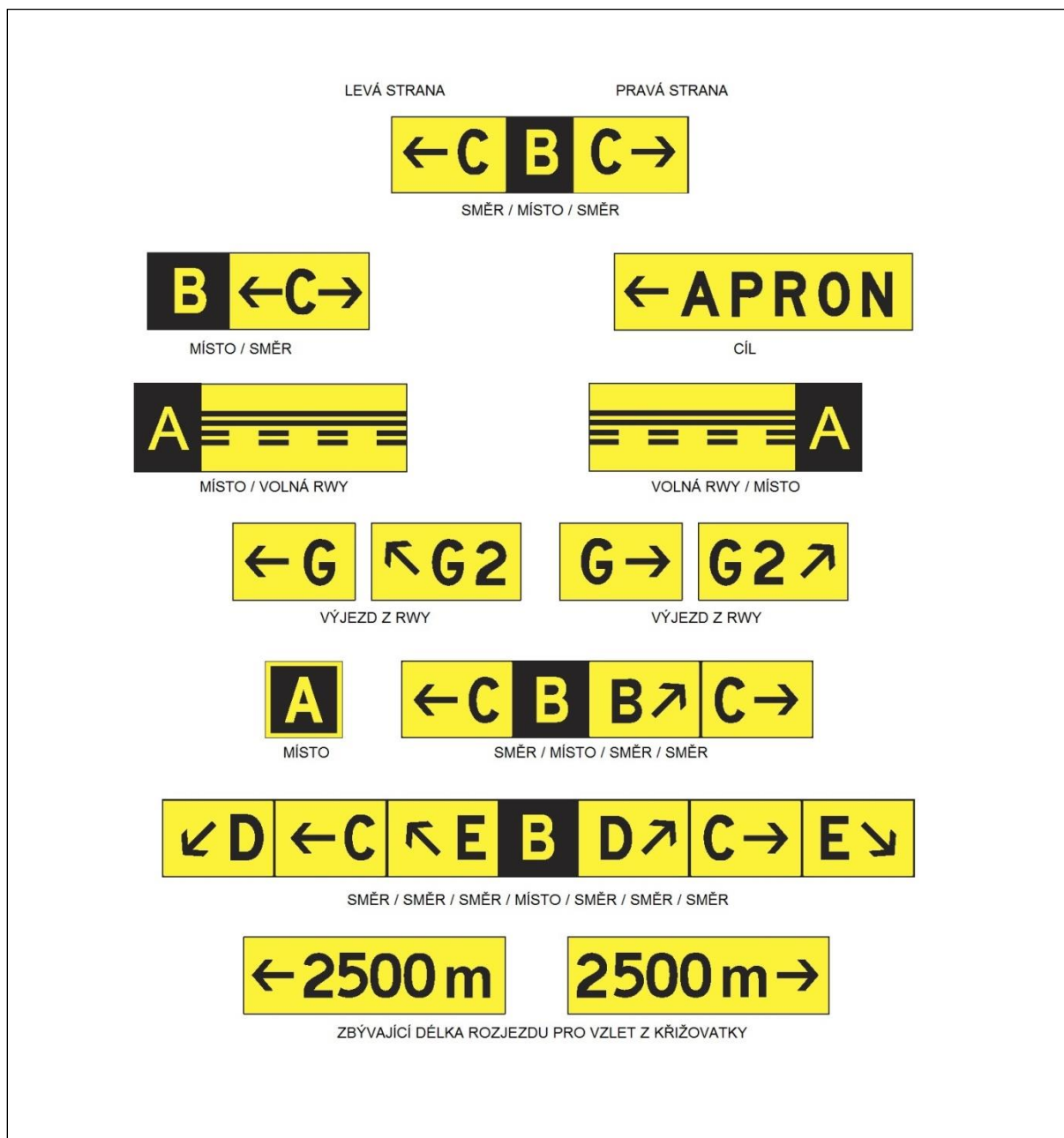
Obrázek N-6. Informační znaky
