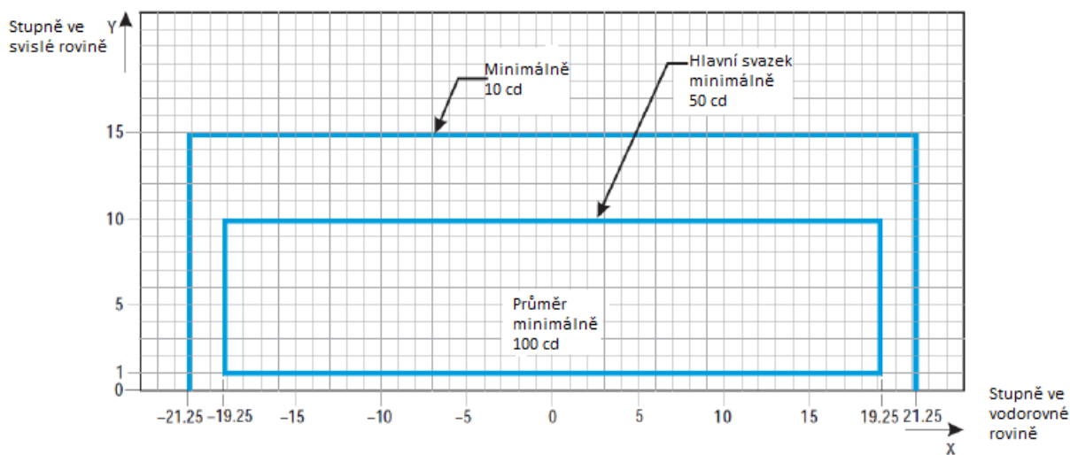
Obrázek U-18. Izokandelový diagram pro osová návěstidla pojezdové dráhy (rozstup 7,5 m), návěstidla REL, příček zákazu vstupu a stop příček v obloucích zatáček určený pro použití v podmínkách RVR nižší než o hodnotě 300 m
