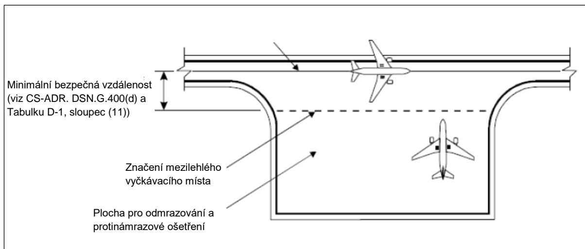
Obrázek G-1. Minimální bezpečné vzdálenosti na ploše pro odmrásování a protinámrazové ošetření
