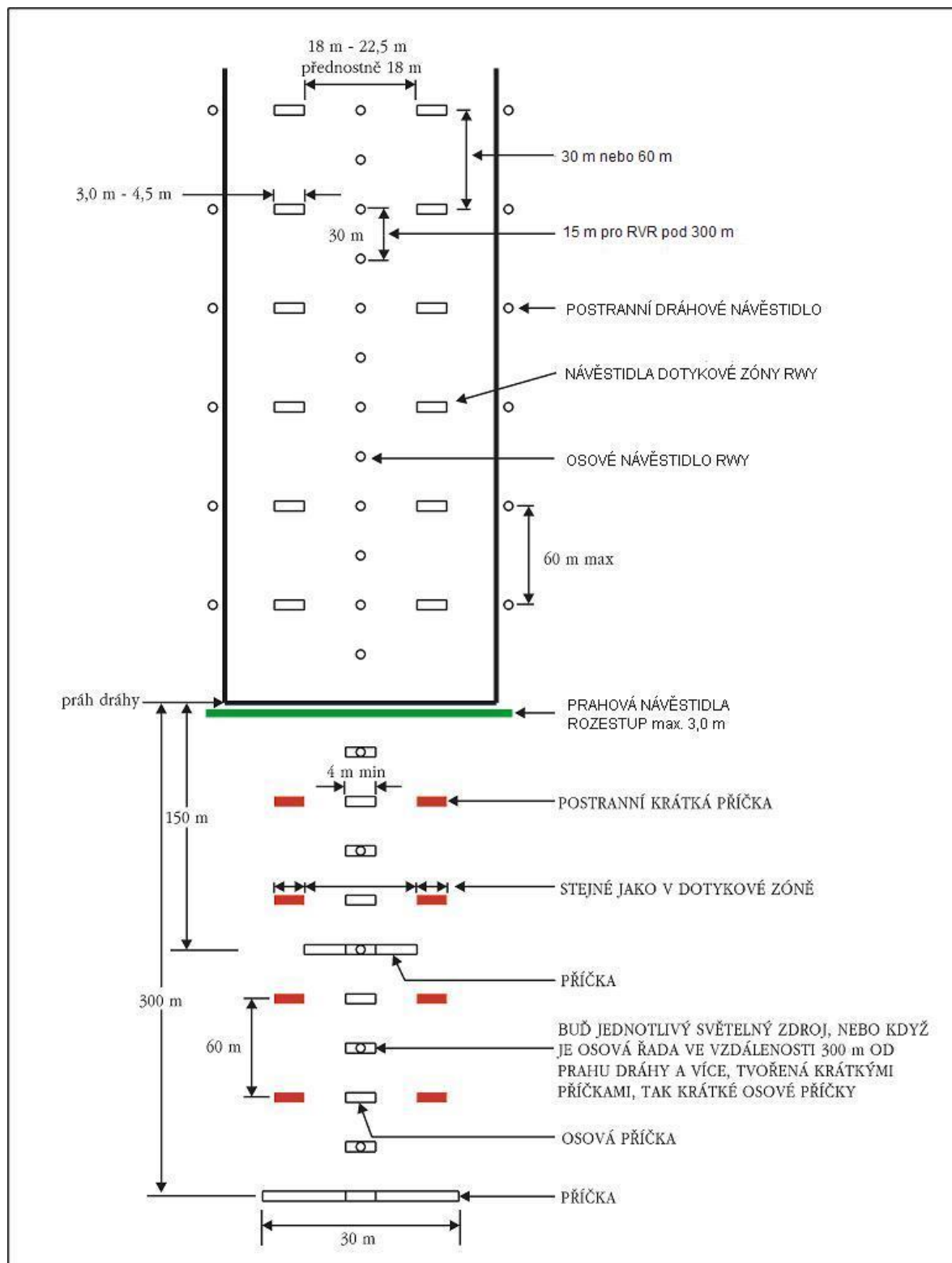
Obrázek M-3B. Vnitřních 300 m světelné přibližovací a dráhové soustavy pro RWY pro přesné přiblížení II. a III. kategorie, když může být prokázána úroveň údržby návestidel splňující požadavky CS ADR-DSN.S.895
