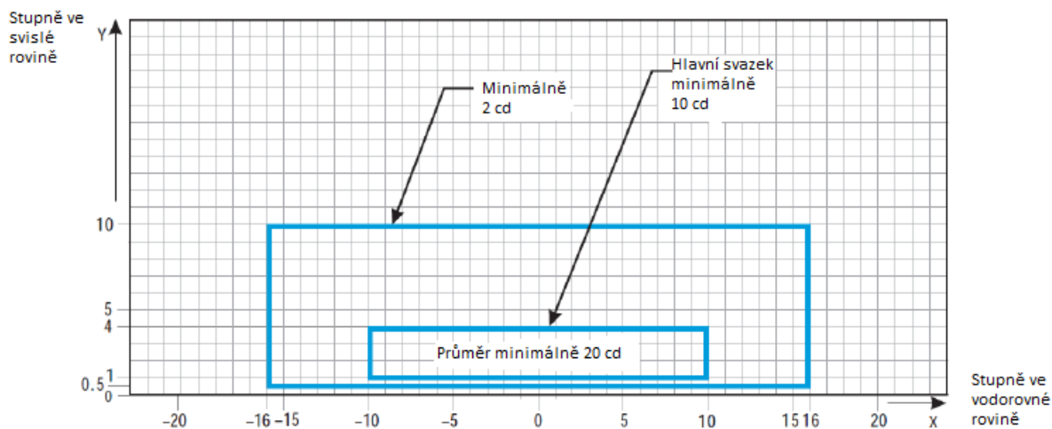
Obrázek U-19. Izokandelový diagram pro osová návěstidla pojezdové dráhy (rozstup 30 a 60 m), příček zákazu vstupu a stop příček v přímých částech určených pro použití v podmínkách RVR 350 m a více
