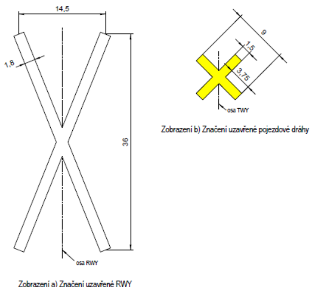
Obrázek R-1. Značení uzavření RWY a pojezdové dráhy
