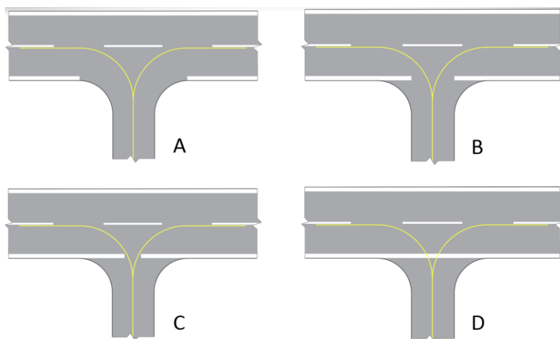
Obrázek GM-L-2. Znárodnění přerušování postranního dráhového značení
