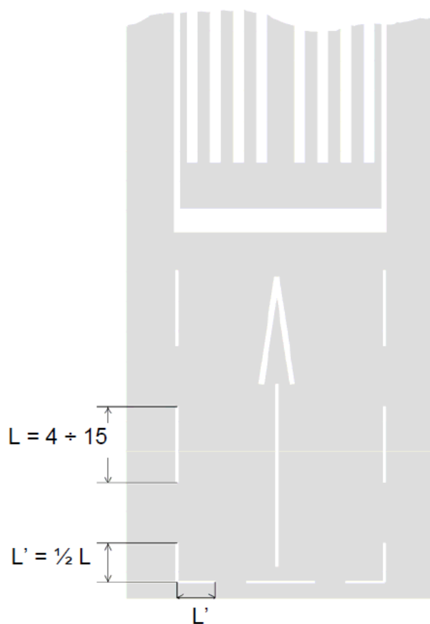
Obrázek GM-L-1. Přerušované značení postranního pásu RWY
