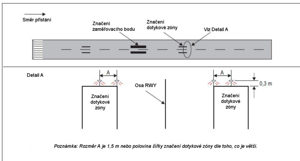
Obr. M-8(C). Jednoduchá návěstidla dotykové zóny
