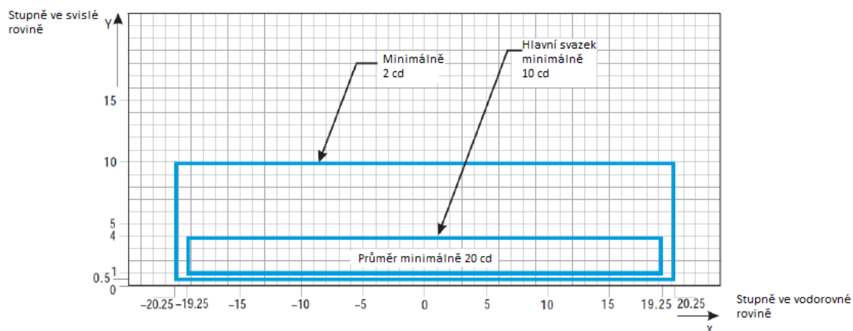
Obrázek U-20. Izokandelový diagram pro osová návěstidla pojezdové dráhy (rozstup 7,5m, 15 m a 30 m), příček zákazu vstupu a stop příček v obloučích zatáček určených pro použití v podmínkách RVR 350 m a více
