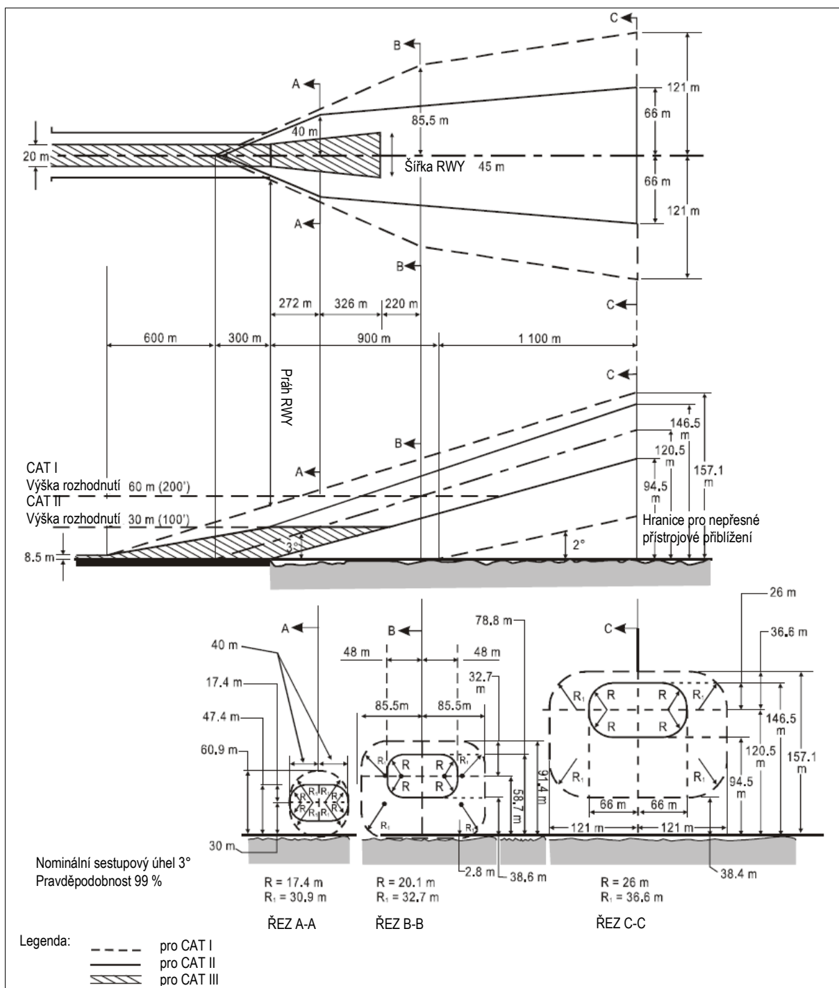
Obrázek GM-M-2. Příklad obálek sestupové dráhy letu pro účely návrhu přibližovací světelné soustavy pro provoz CAT I, II a III – osová návěstidla
