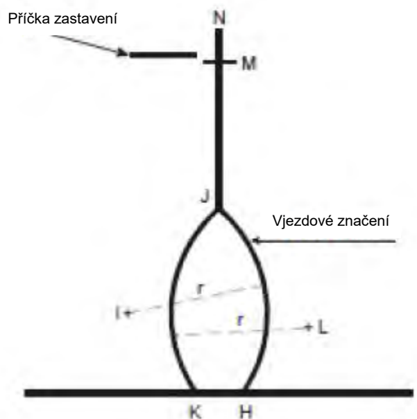
Obrázek 9 – Posunuté vjezdové značení příďového podvozku
