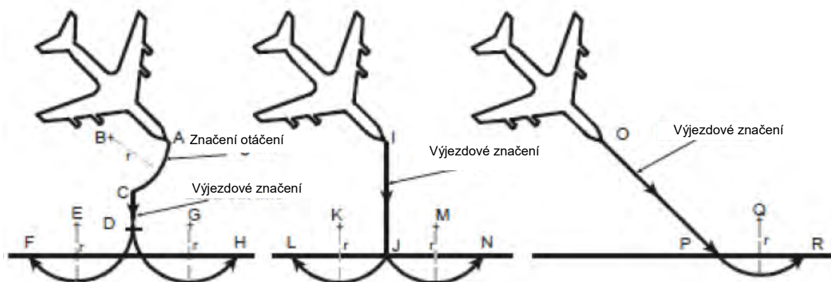
Obrázek 11 – Posunuté výjezdové značení příďového podvozku
