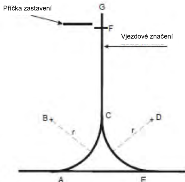
Obrázek 8 – Jednoduché vjezdové značení příďového podvozku
