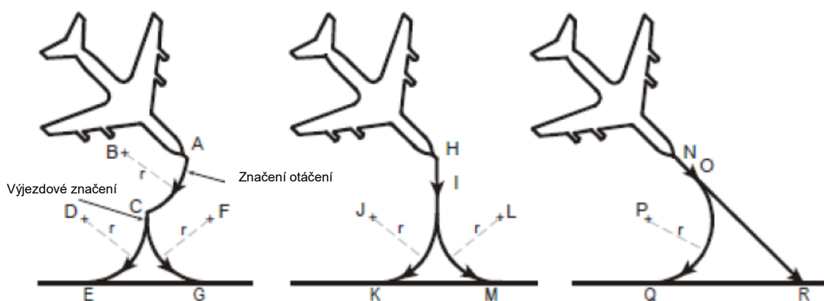
Obrázek 10 – Jednoduché vjezdové značení příďového podvozku
